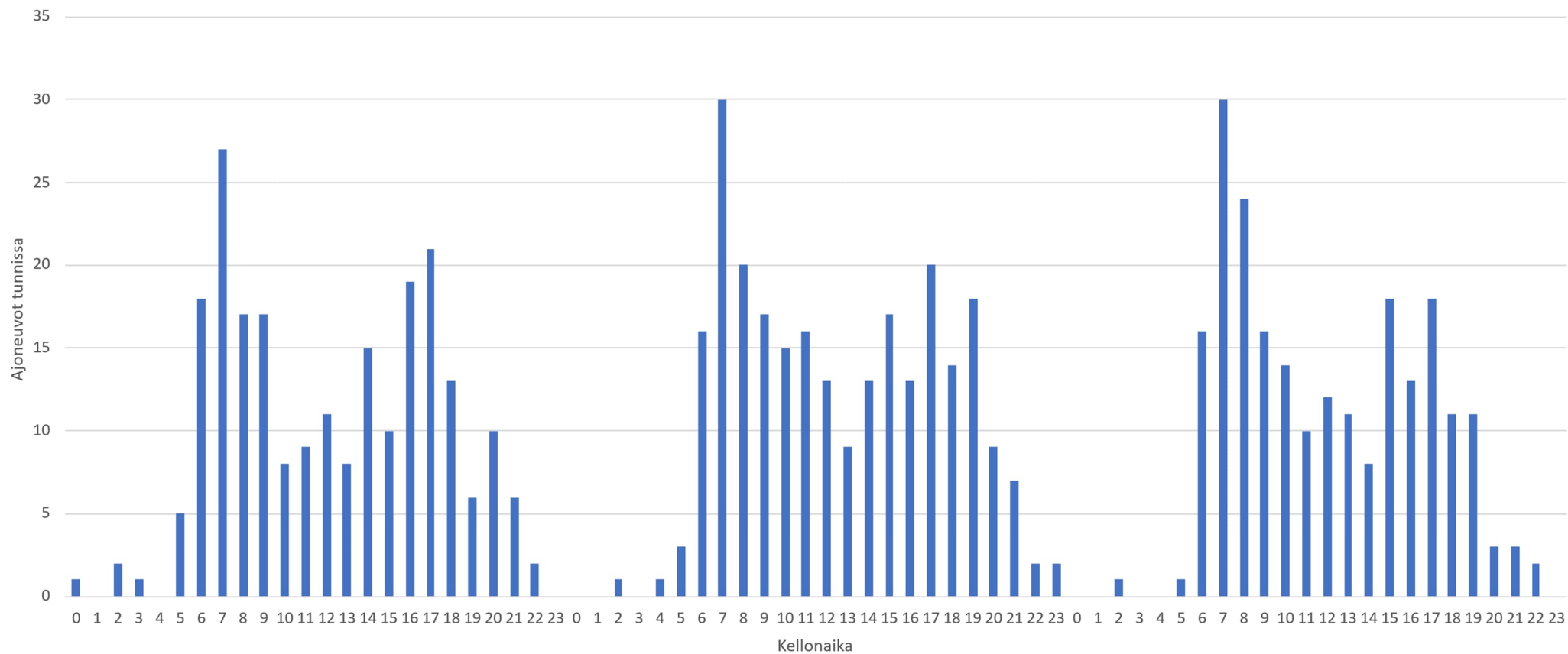
Liikennetiedot ajoneuvoryhmittäin, 13.01.–15.01.2026, Piste 2 Suunta B
