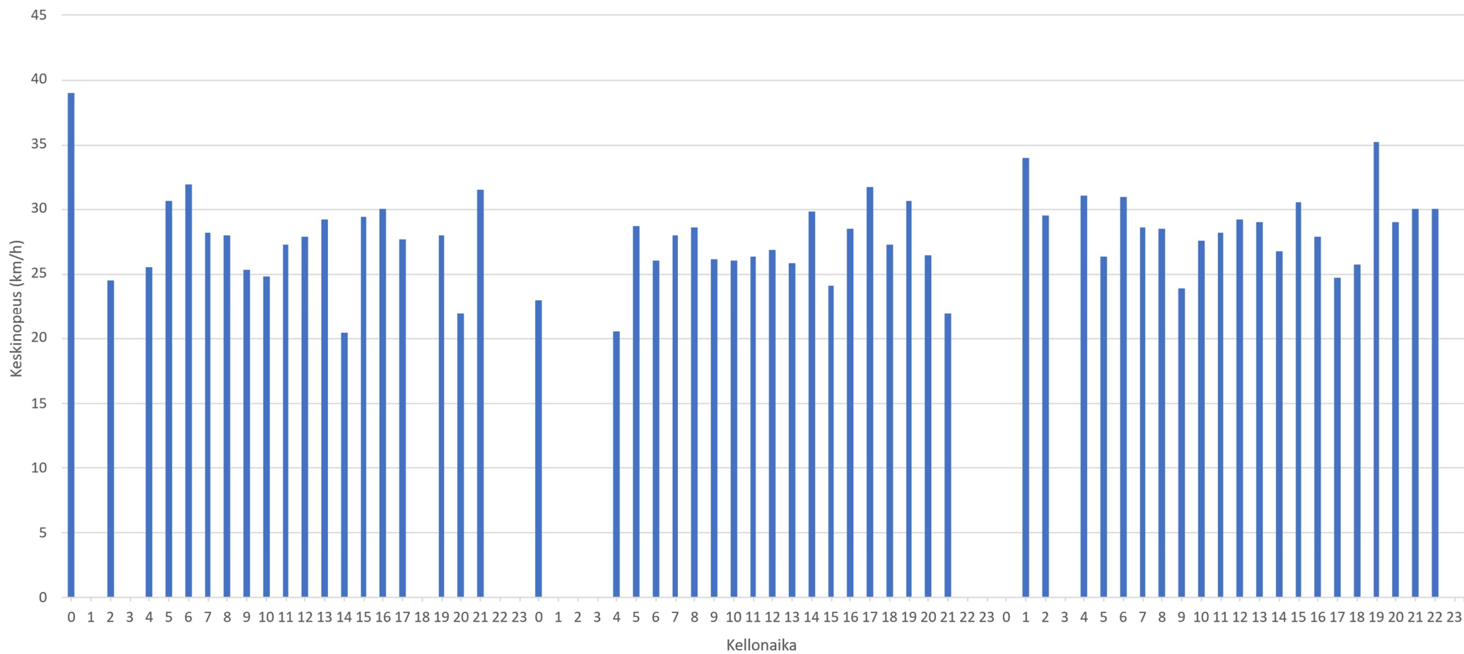
Tuntikohtainen keskinopeus (km/h), 13.01.—15.01.2026, Piste 1 Suunta A
