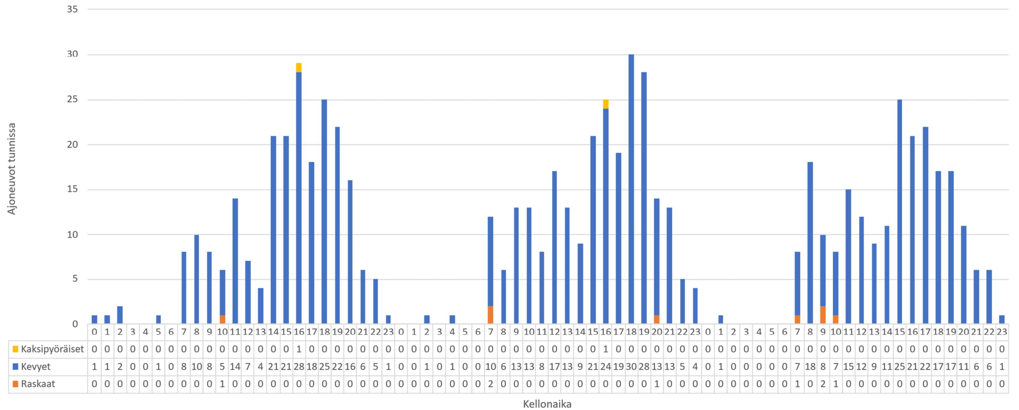
Liikennetiedot ajoneuvoryhmittäin, 13.01.—15.01.2026, Piste 2 Suunta A
