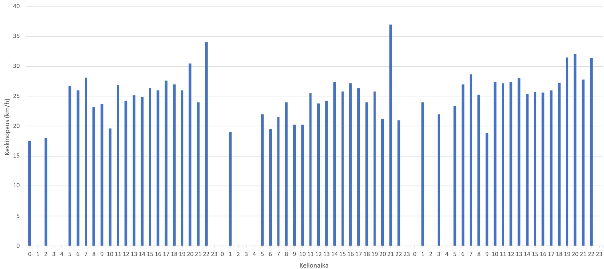
Tuntikohtainen keskinopeus (km/h), 13.01.—15.01.2026, Piste 1 Suunta B
