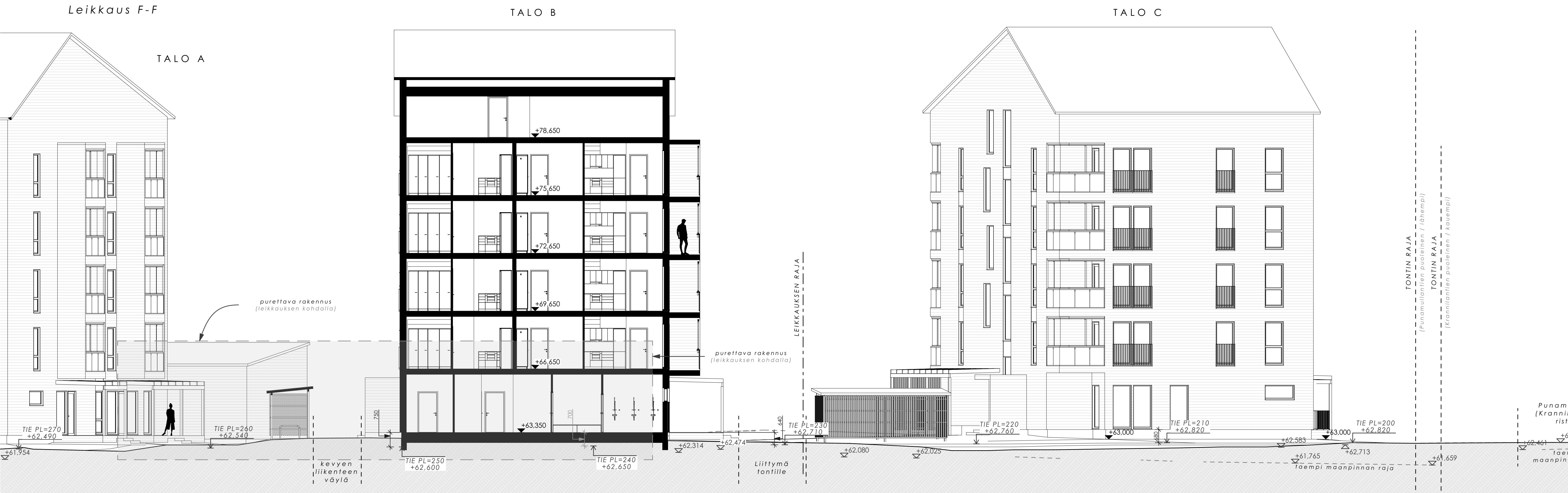
Leikkaus F-F
