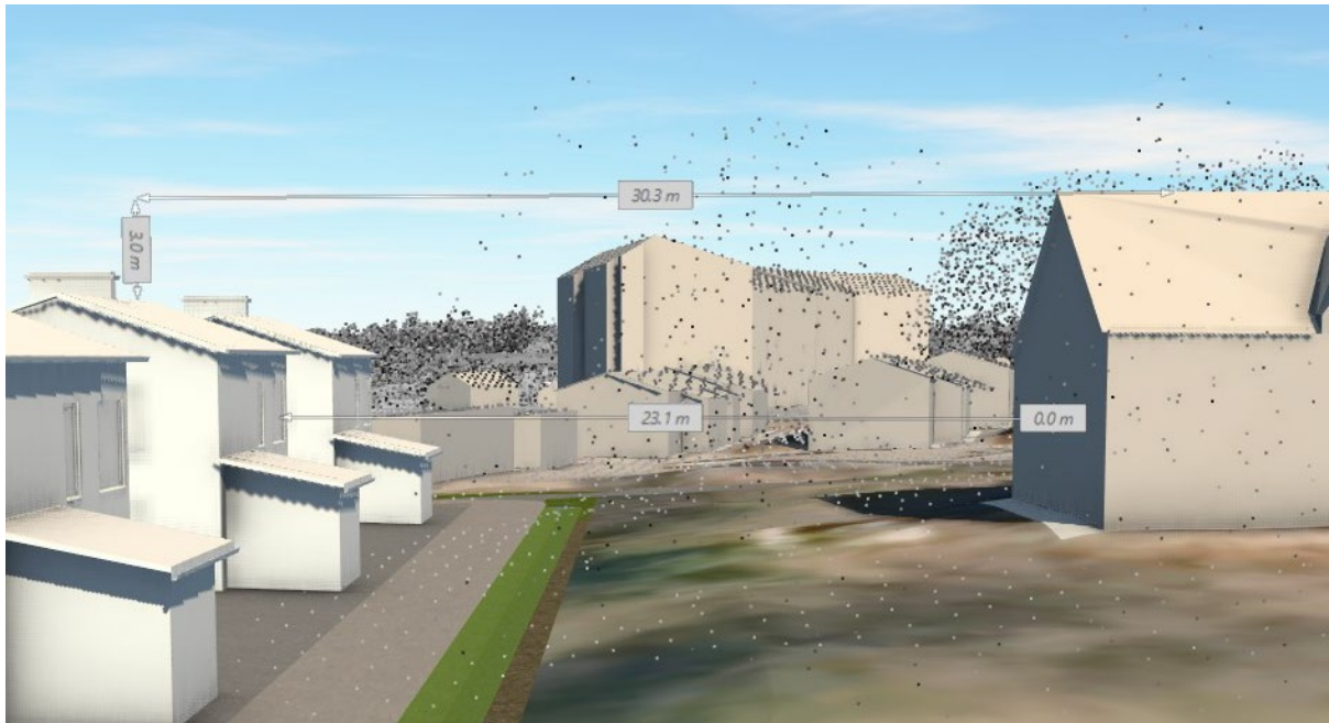
Kuva 3 mittaukset kattotarhojen ja kerrosten korkeusasemista. Pistepilvi osoittaa välissä olevan nykyisen puuston.
