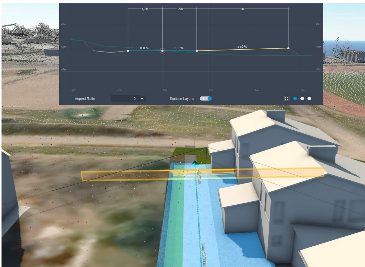
Kuva 4 pihan mittauksia. Etäisyys tontinrajasta esimerkinomaisen rakennusten välissä sijaitsevan autokatoksen seinään on 9 m, jolloin tontilla voidaan kääntyä autokatokseen. Suunnitelma voidaan toteuttaa toisillakin tavoilla, esimerkiksi pitkittäisillä autokatoksilla rajan suuntaisesti.
