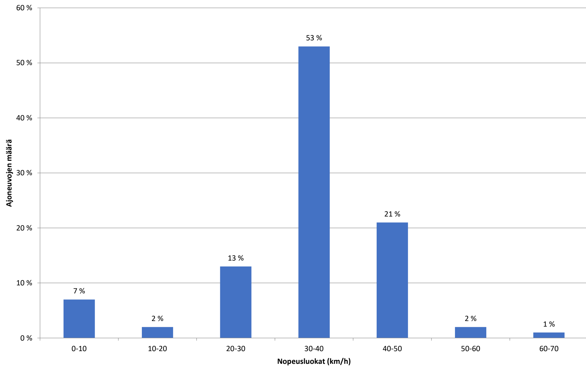
Piste 3 B Nopeusjakauma - Koko mittaus
