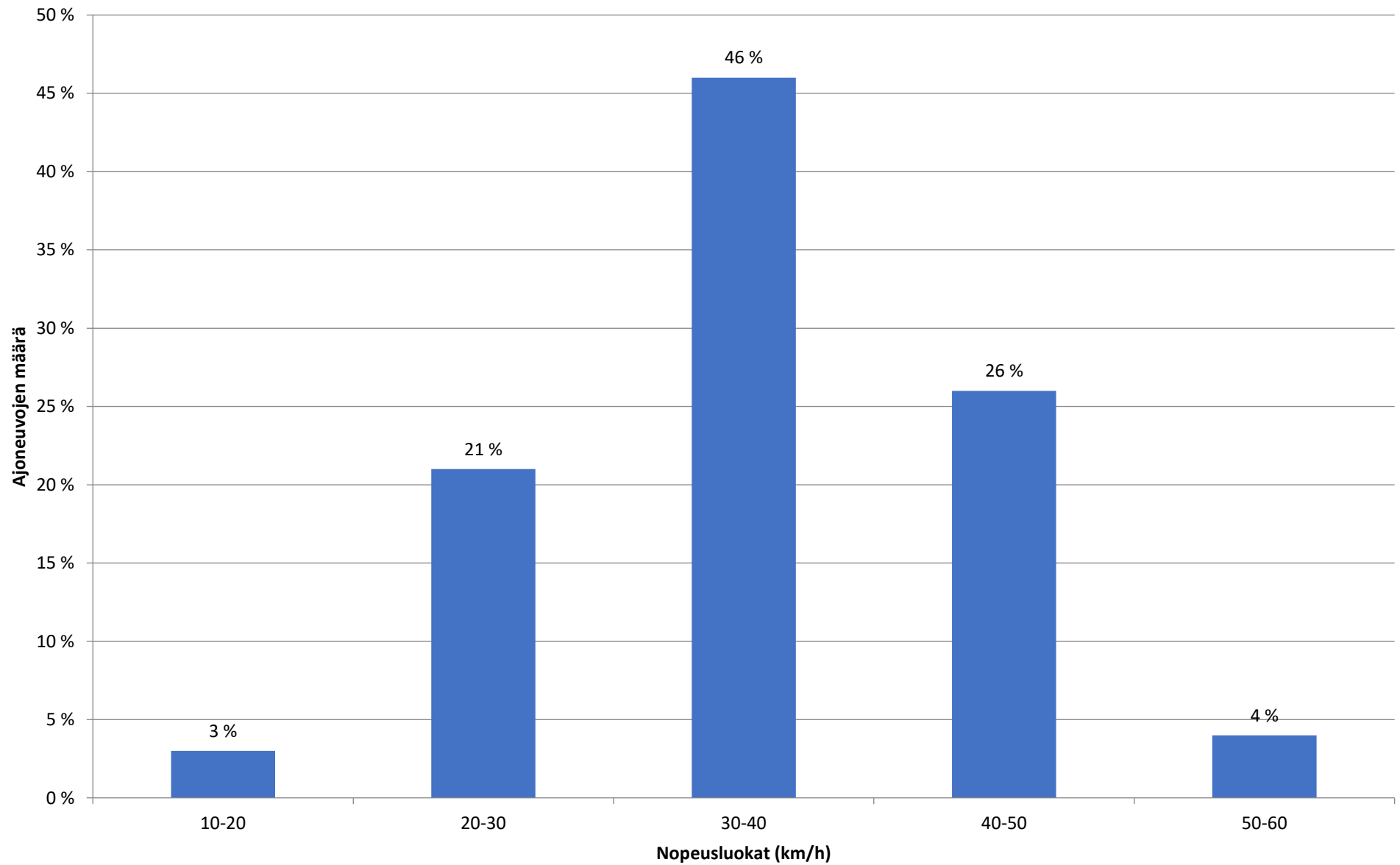
Piste 2 A Nopeusjakauma - Koko mittaus
