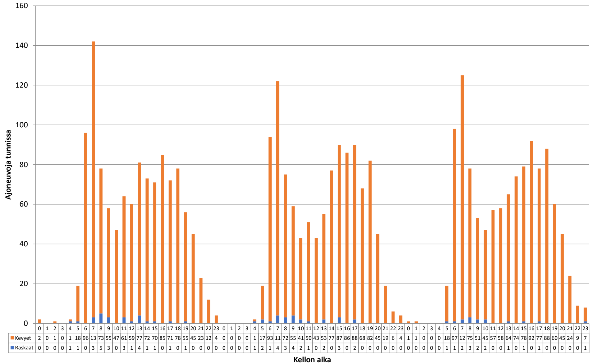
Piste 2 B Liikennetiedot ajoneuvoryhmittäin - 20.11.2018-22.11.2018
