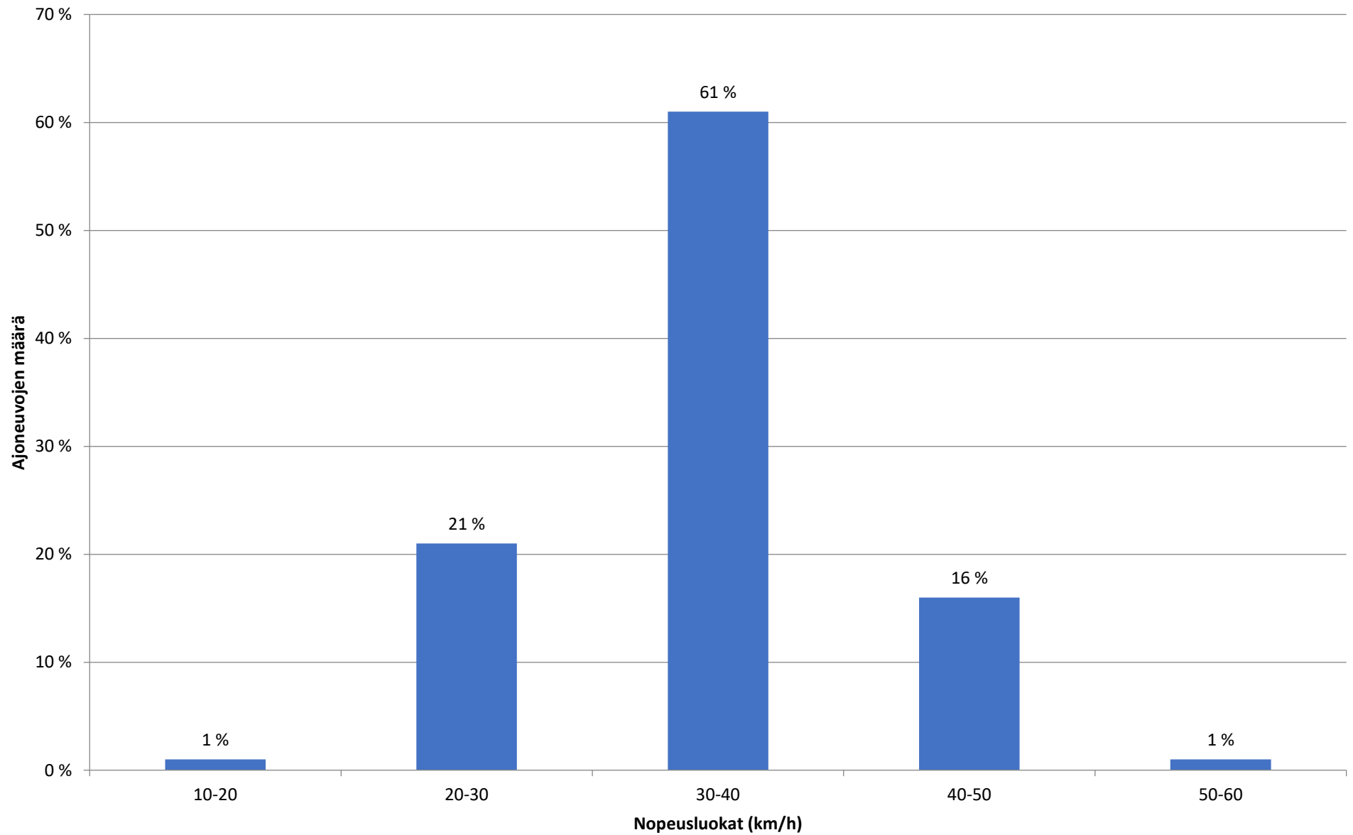
Piste 5 Nopeusjakauma - Koko mittaus
