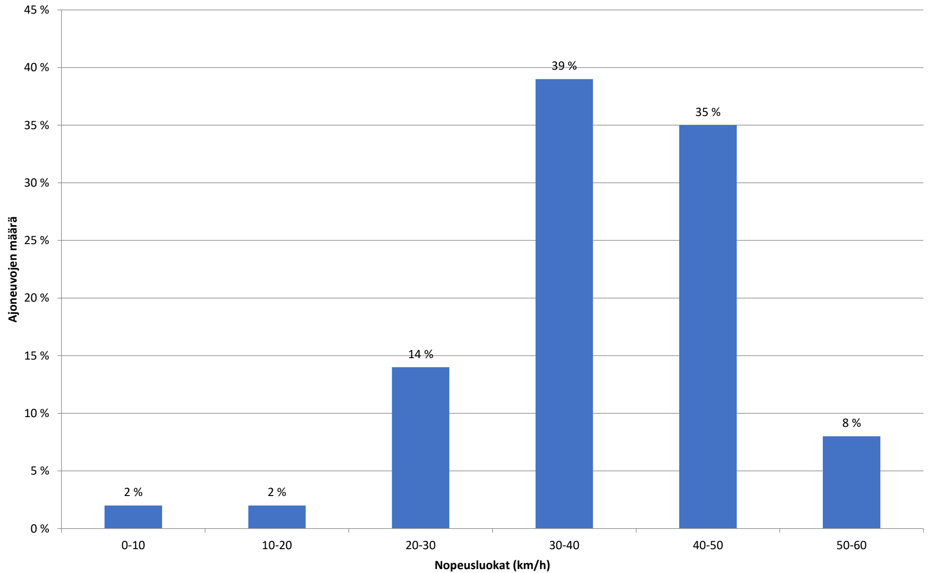
Piste 1 B Nopeusjakauma - Koko mittaus
