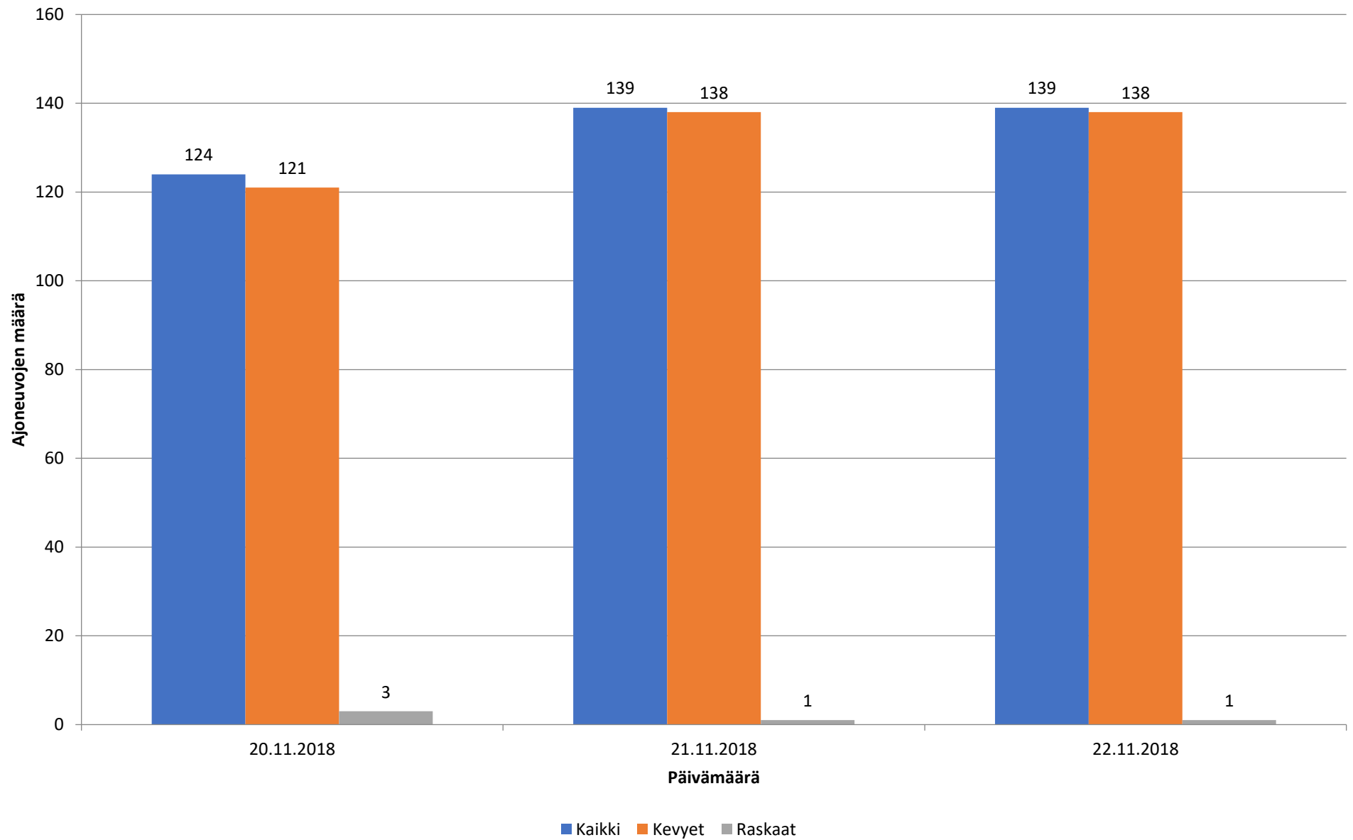
Piste 3 A Liikennetiedot ajoneuvoryhmittäin
