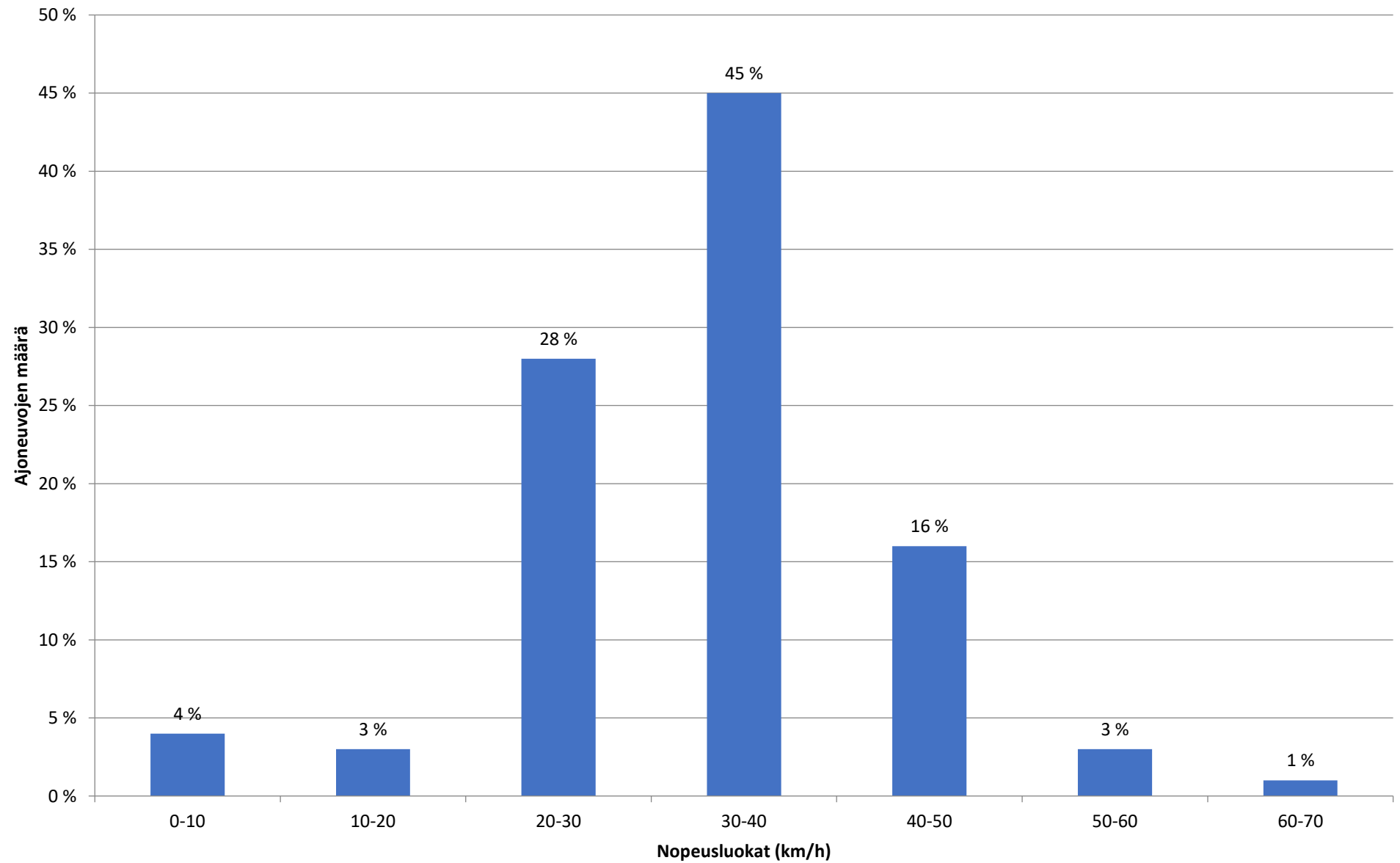
Piste 1 A Nopeusjakauma - Koko mittaus
