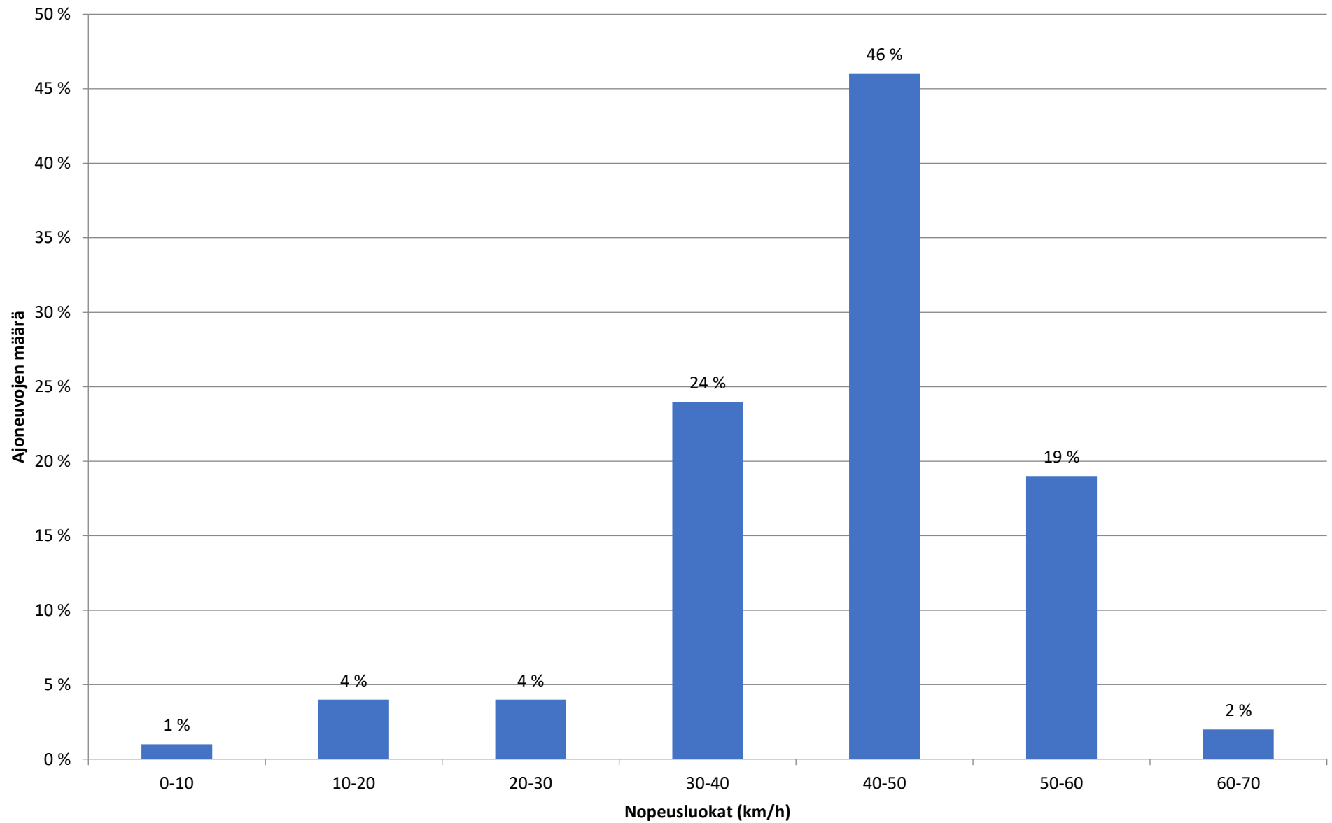
Piste 6 A Nopeusjakauma - Koko mittaus
