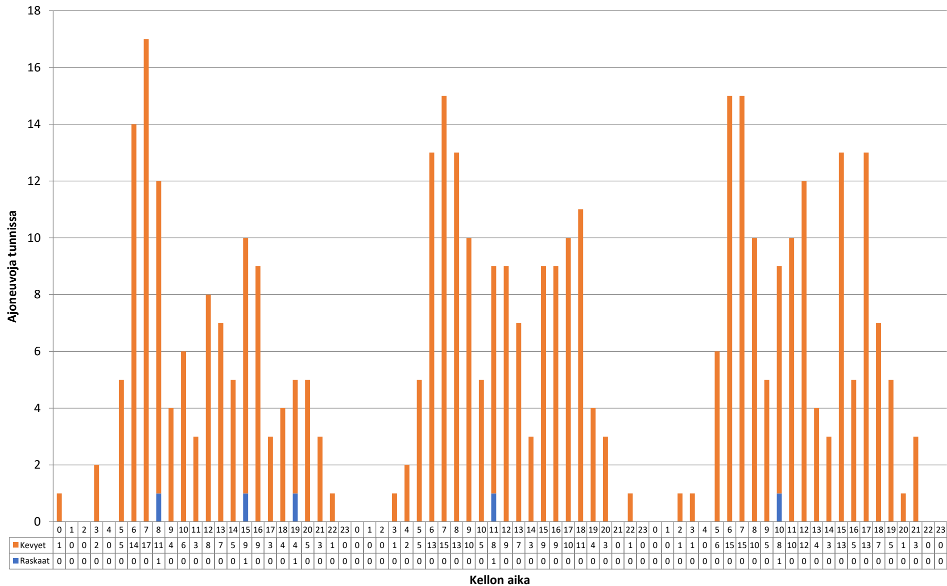
Piste 3 A Liikennetiedot ajoneuvoryhmittäin - 20.11.2018-22.11.2018
