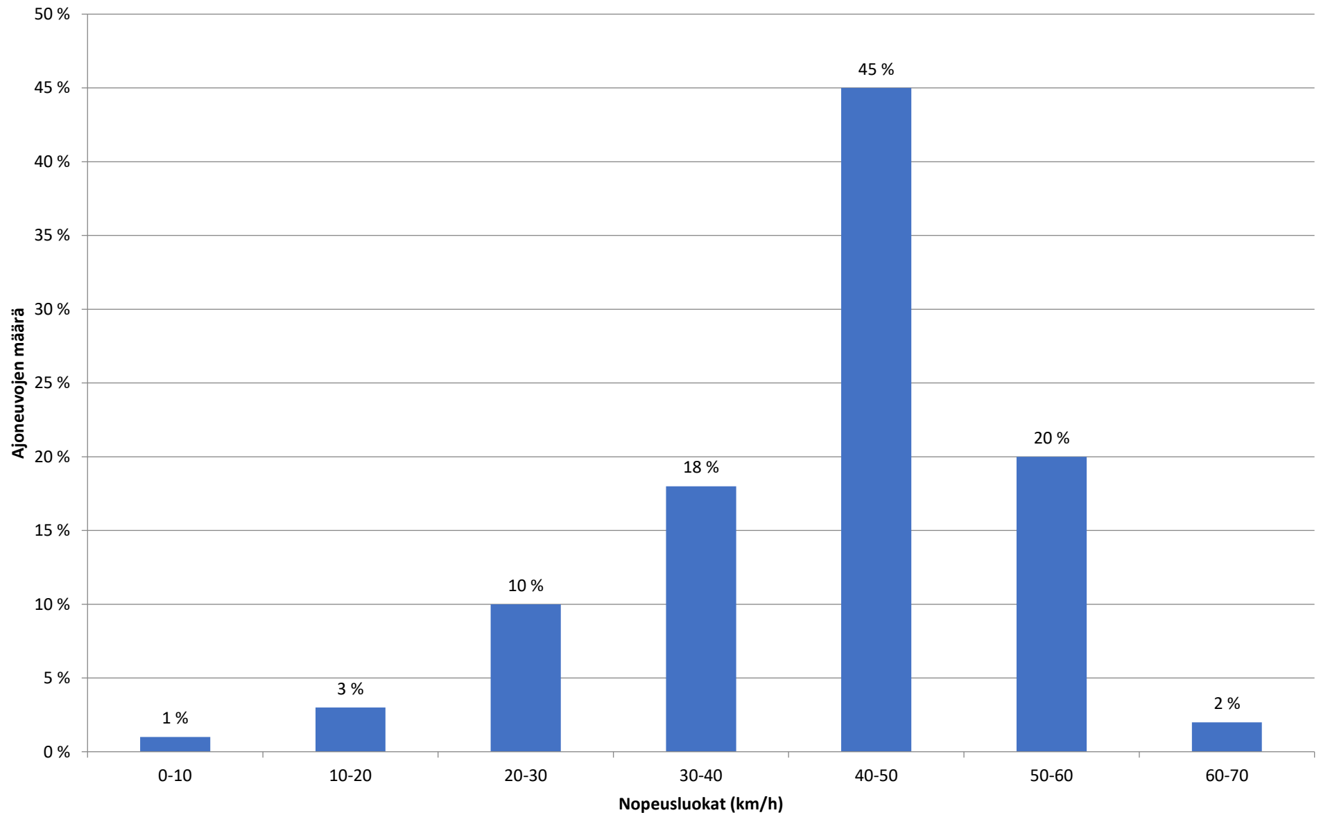
Piste 6 B Nopeusjakauma - Koko mittaus
