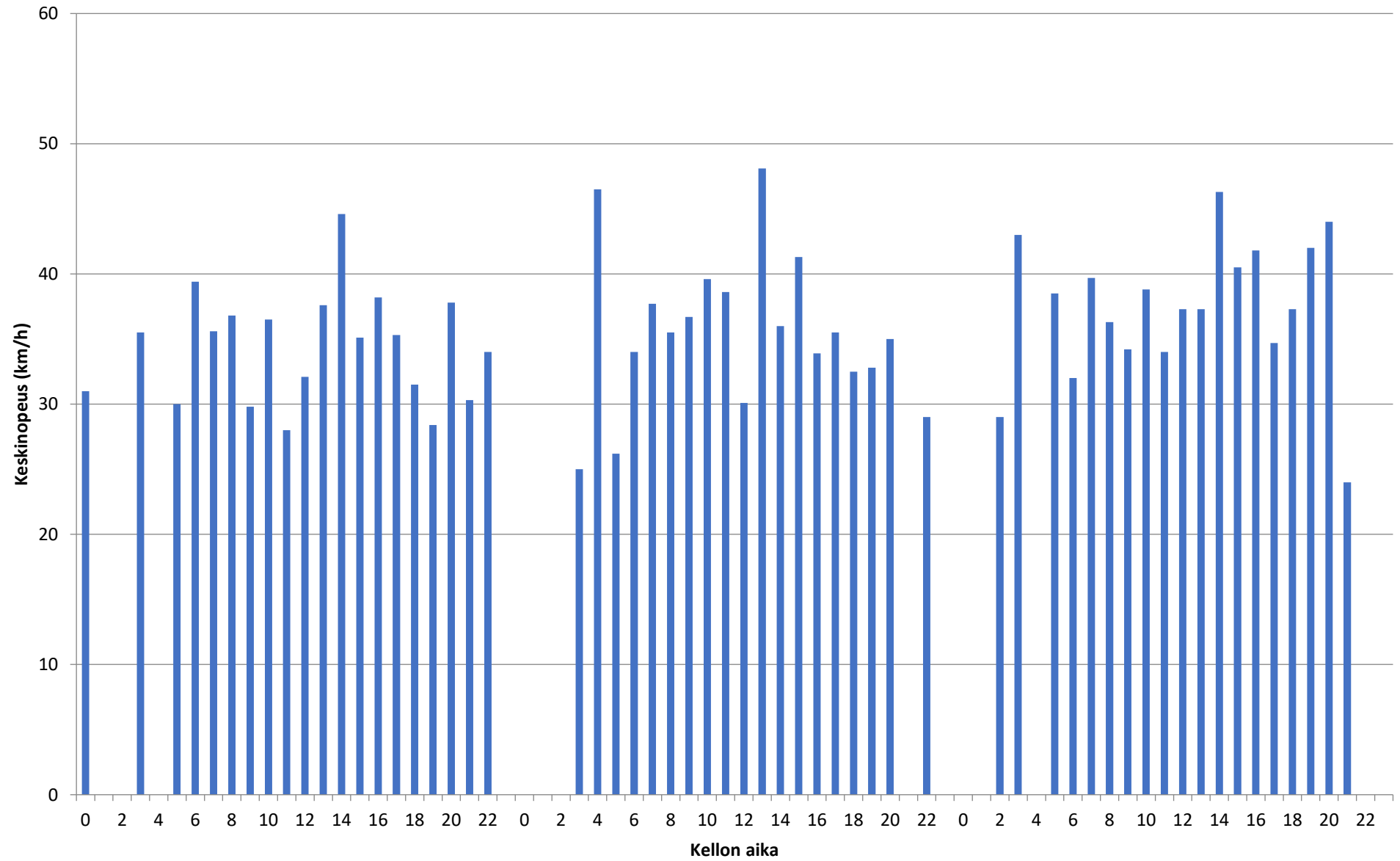
Piste 3 A Keskinopeus - 20.11.2018-22.11.2018
