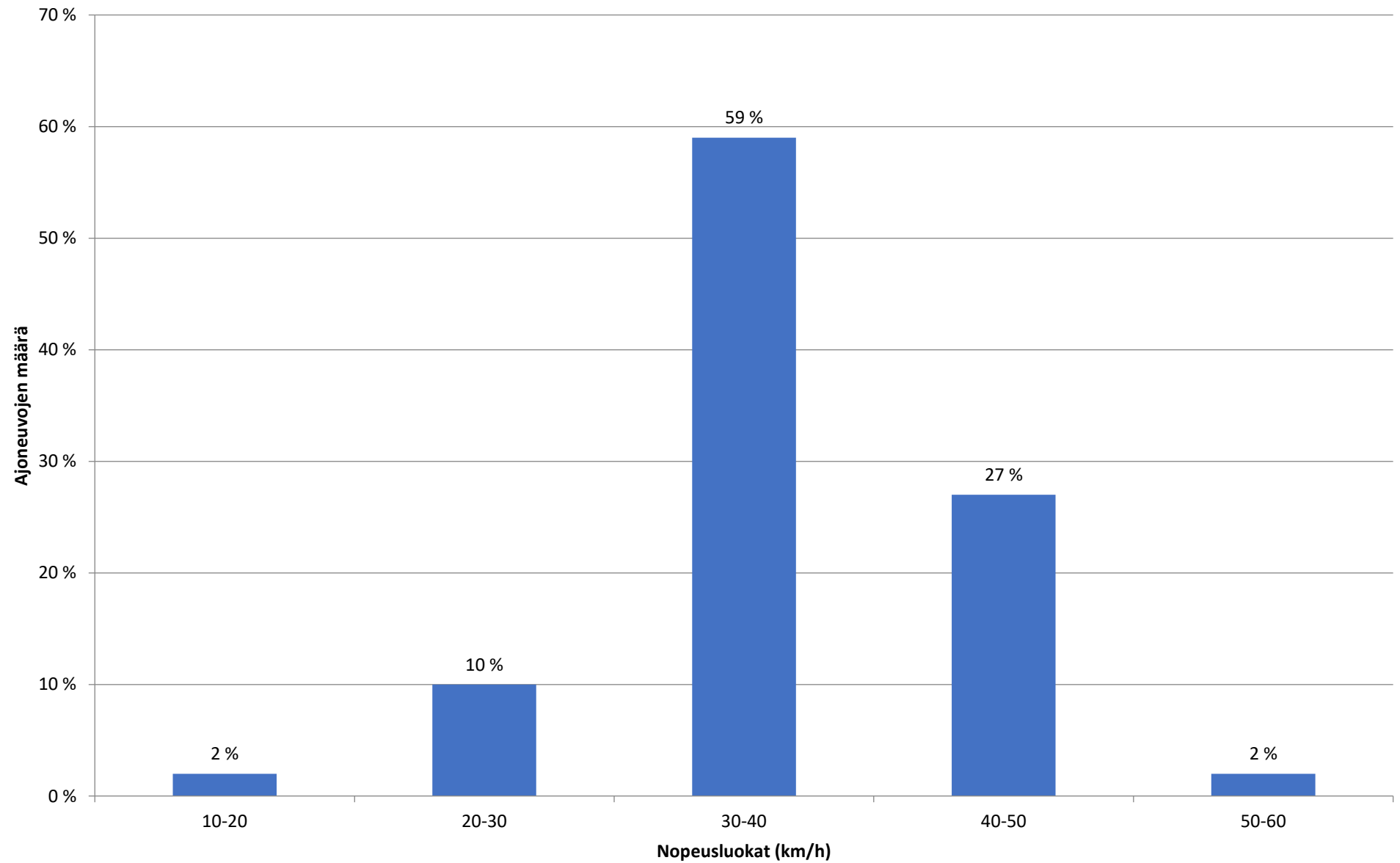
Piste 4 Nopeusjakauma - Koko mittaus
